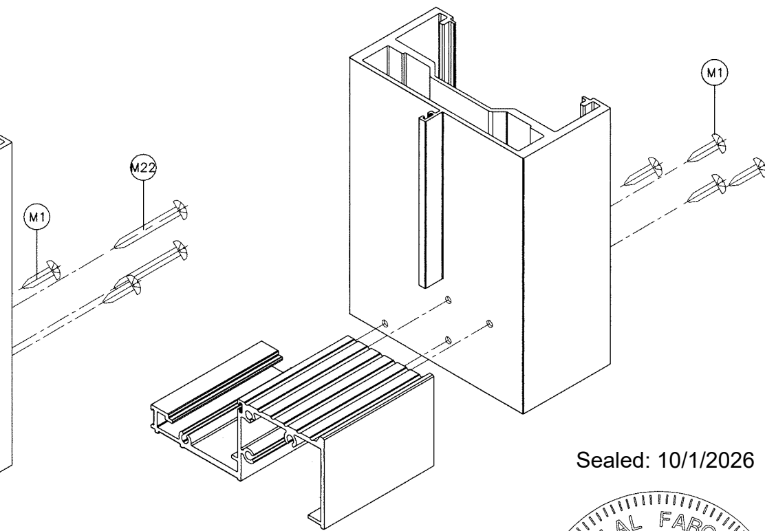
FRAME BOTTOM CORNER STD. JAMB
